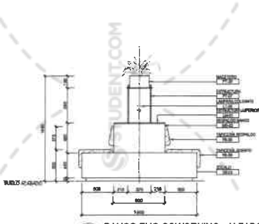
BANCO FIJO COWORKING - ALZADO LATERAL SCALE 1:20
