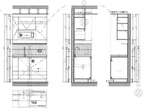
DETALLE MUEBLE DE COCINA C2
