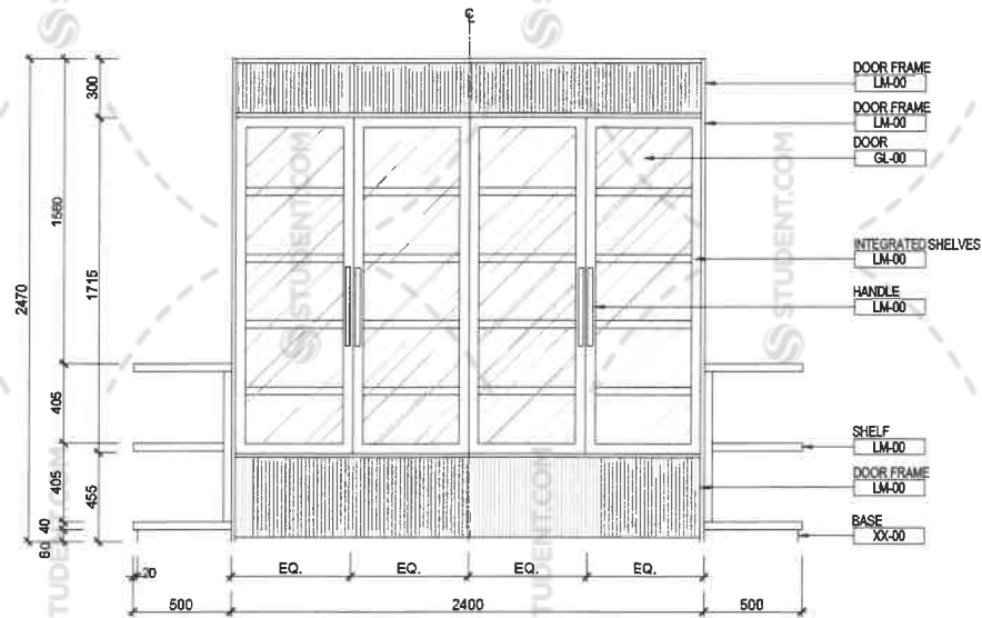
3 IDG-5.04 MINI MARKET FRIDGE - ELEVATION SCALE 1:20
