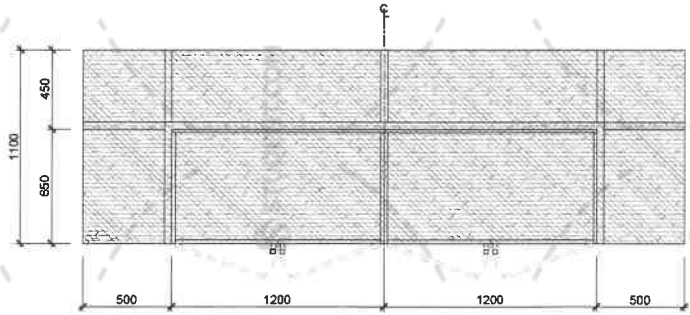
2 IDG-5.04 MINI MARKET FRIDGE - SECTION PLAN SCALE 1:20
