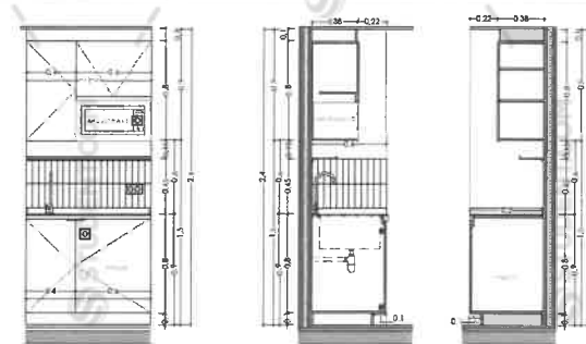
DETALLE MUEBLE DE COCINA C1
