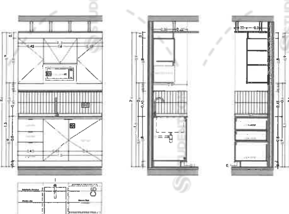
DETALLE MUEBLE DE COCINA C6
