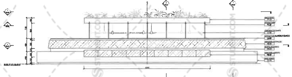
BANCO FIJO COWORKING - ALZADO SCALE 1:20
